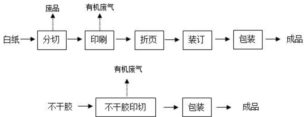
图 3-3 本项目生产工艺流程图
