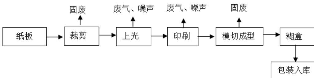
图 3-3 本项目生产工艺流程图
