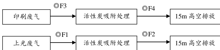
图 4-2 废气处理工艺流程图
