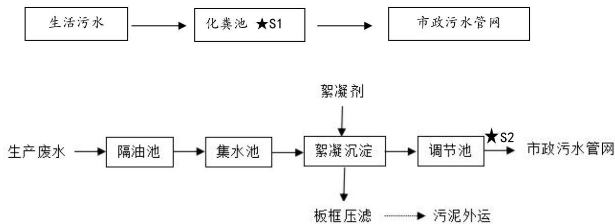
图 4-1 废水处理工艺流程图
