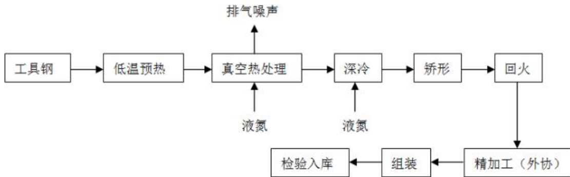
图 3-3 本项目生产工艺流程图
