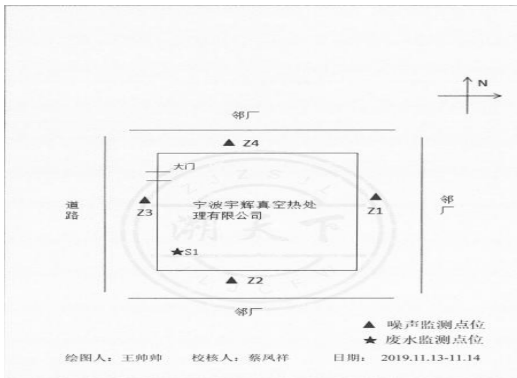
图 7-1 监测点位图
