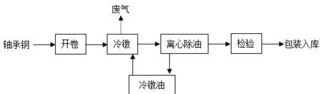
图 3-3 本项目生产工艺流程图
