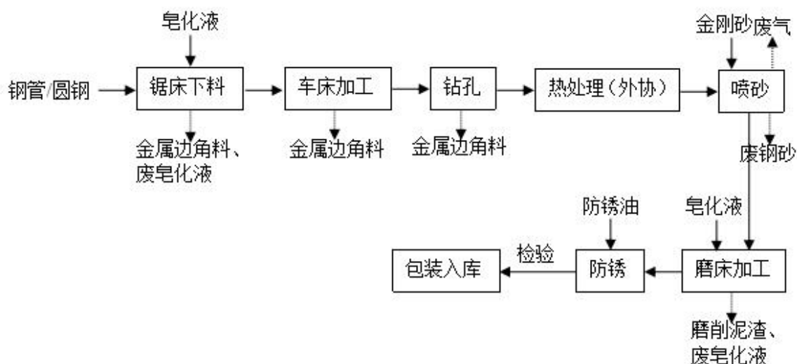
图 3-3 本项目生产工艺流程图
