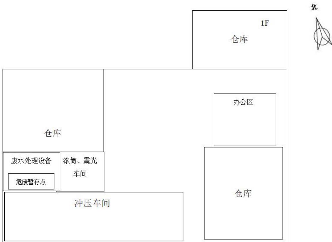
图 3-2 厂区平面布置图
