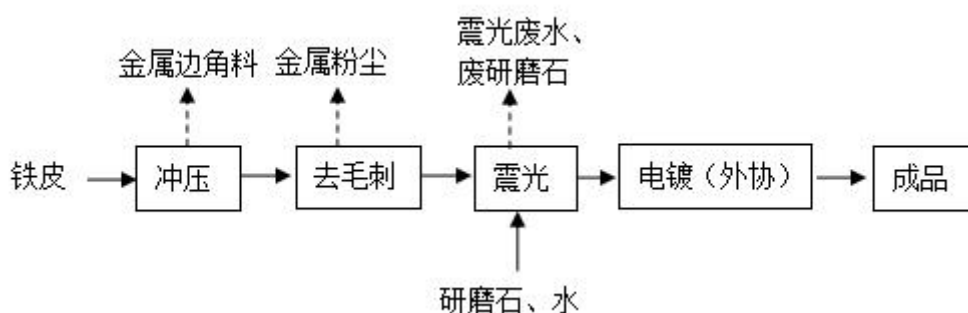
图 3-3 渔具配件生产工艺及产污环节示意图
