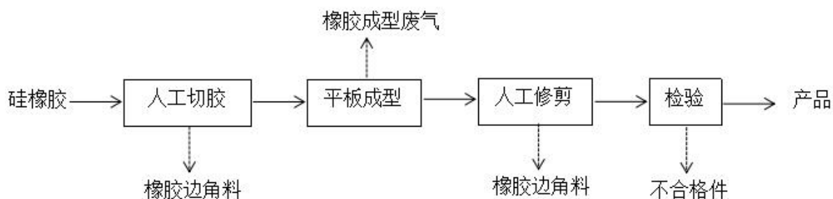
图 3-3 硅胶圈生产工艺及产污环节流程图
