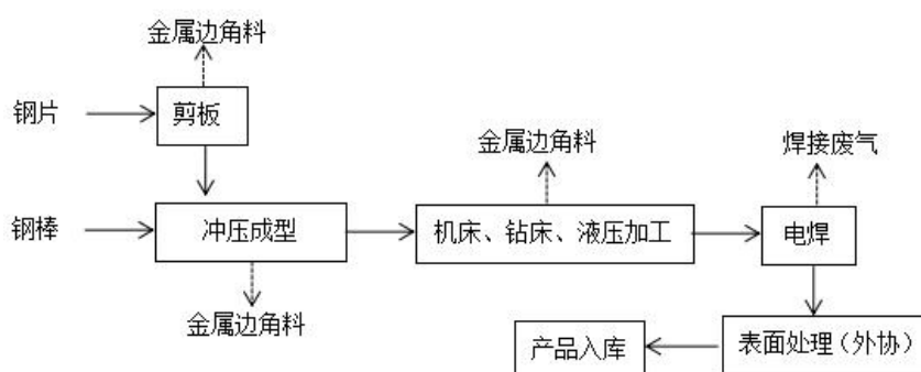
图 3-3 本项目生产工艺流程图
