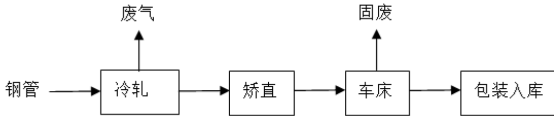
图 3-3 本项目生产工艺流程图
