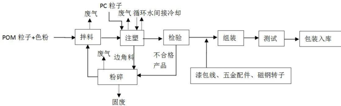
图 3-4 本项目生产工艺流程图
