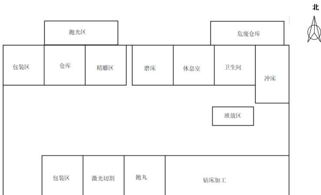
图 3-2 厂区平面布置图（1F）
