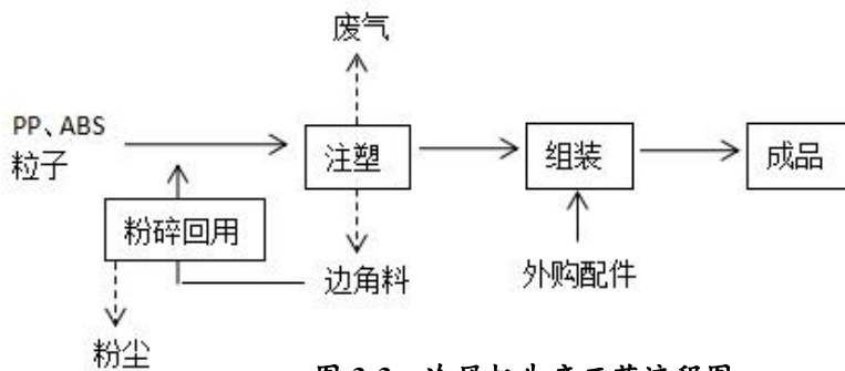
图 3-3 冷风机生产工艺流程图
