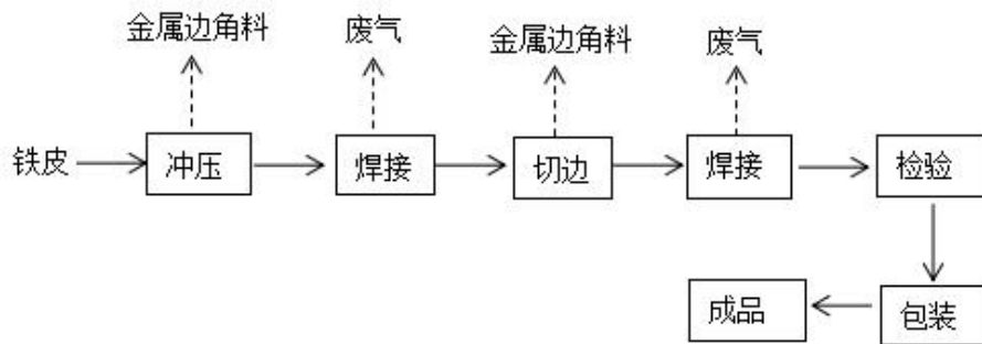
图 3-4 油汀生产工艺流程图
