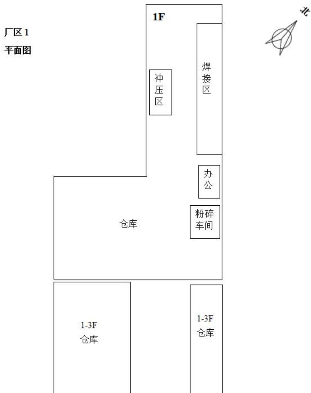
图 3-2 厂区 1 平面布置图 (1F)
