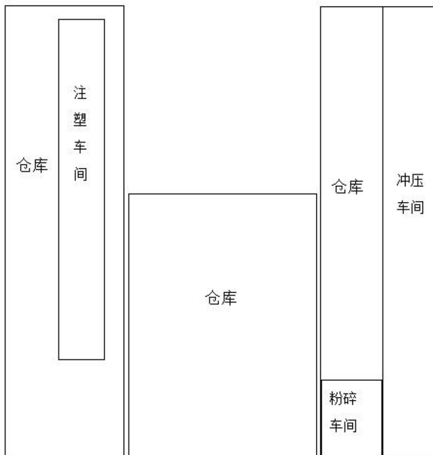
图 3-2 厂区平面布置图 (1F)
