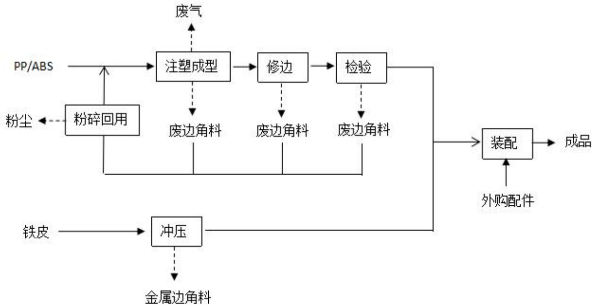
图 3-3 本项目生产工艺流程图
