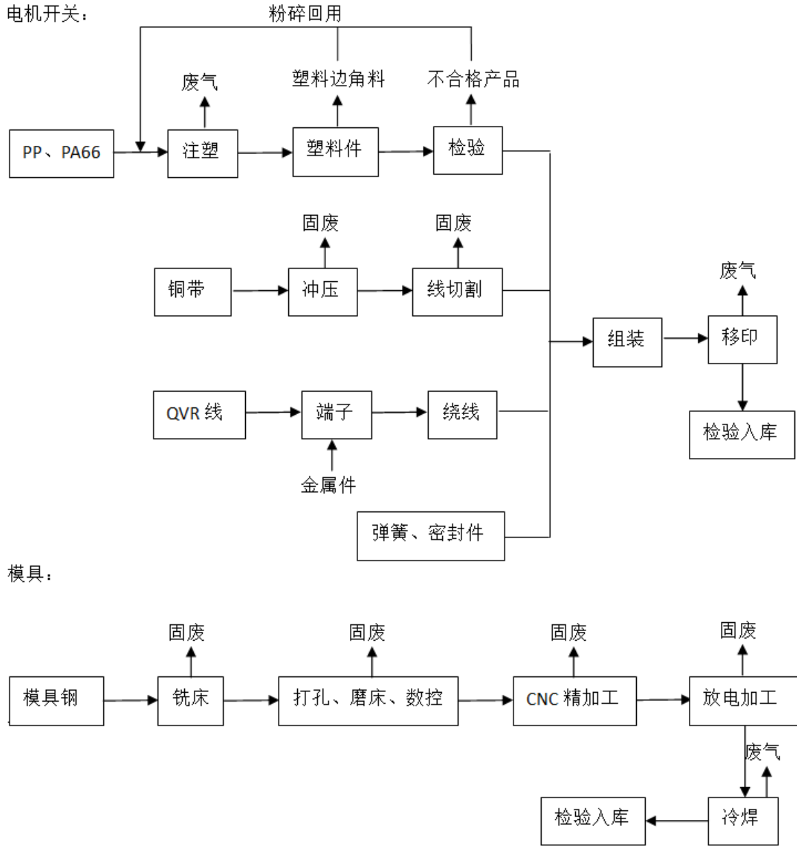
图 3-3 本项目生产工艺流程图
