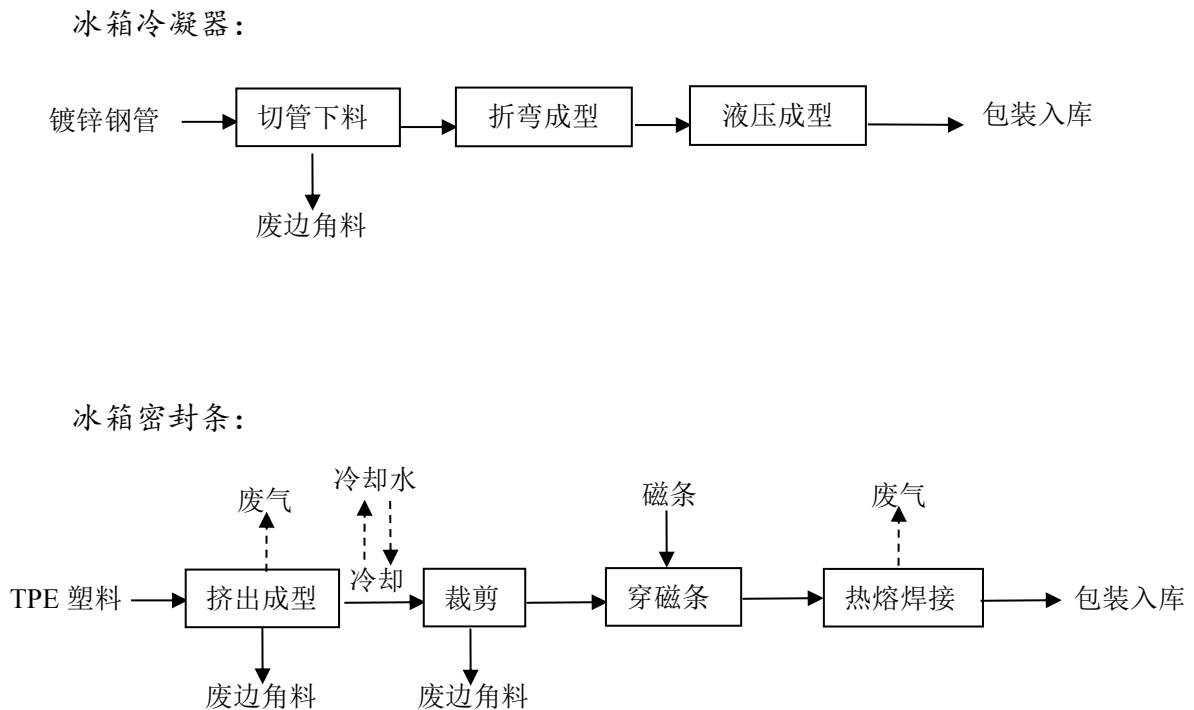
图 3-3 本项目生产工艺流程图
