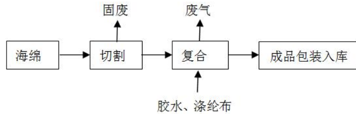
图 3-3 本项目生产工艺流程图
