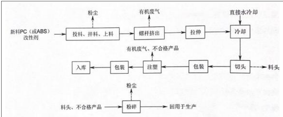
图 2-1 卫浴排水器生产工艺流程及产污节点图
