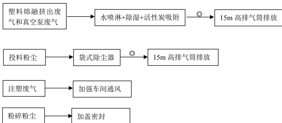
图 3-1 废气处理工艺流程图
