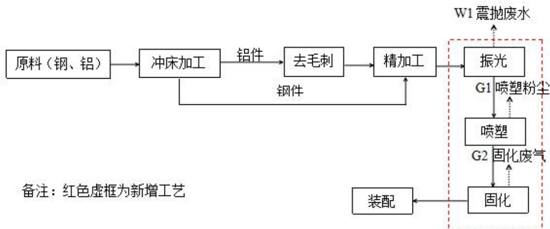
图 3-3 本项目生产工艺流程图
