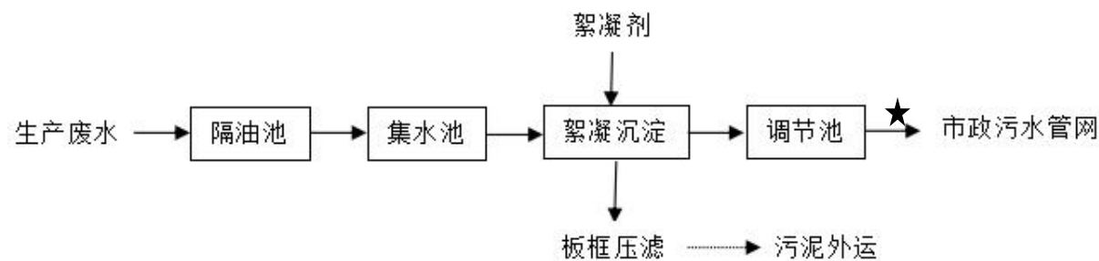
图 4-1 废水处理工艺流程图
