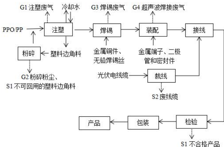
图 2-1 光伏接线盒生产工艺流程图及产污节点图
