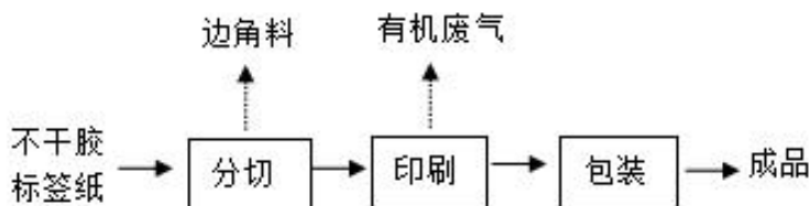
图 3-4 不干胶生产工艺及产污环节流程图
