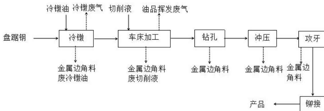
图 3-3 紧固件生产工艺及产污环节流程图
