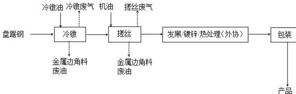
图 2-1 紧固件生产工艺流程及产污节点图
