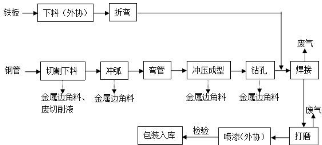
图 2-1 清洗机支架生产工艺流程及产污节点图
