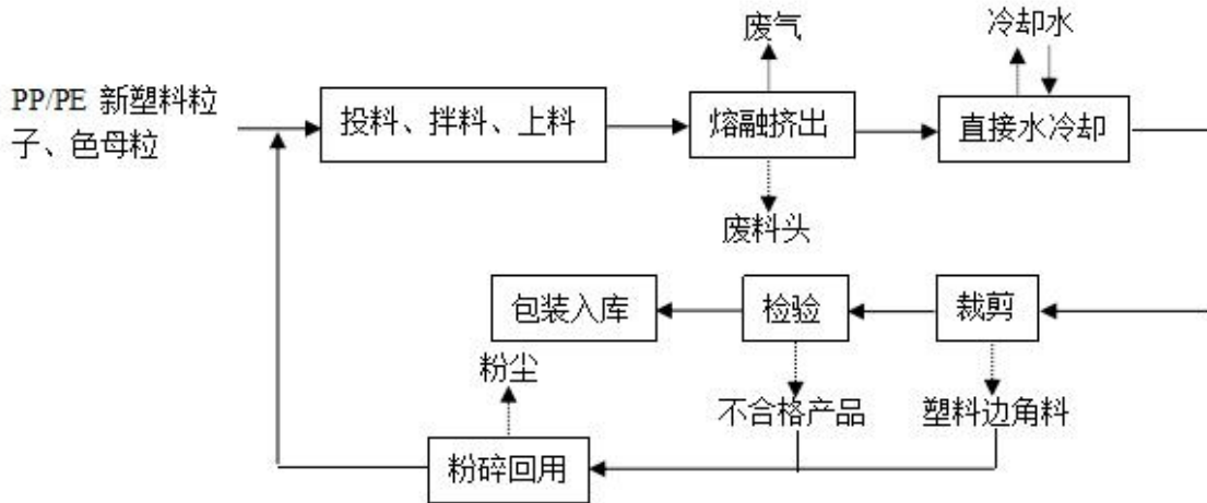
图 2-1 本项目塑料管生产工艺及产污环节流程图
