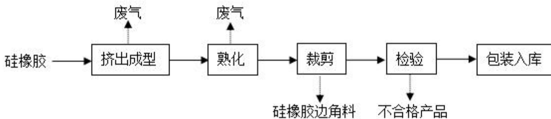
图 2-2 本项目硅胶管生产工艺及产污环节流程图
