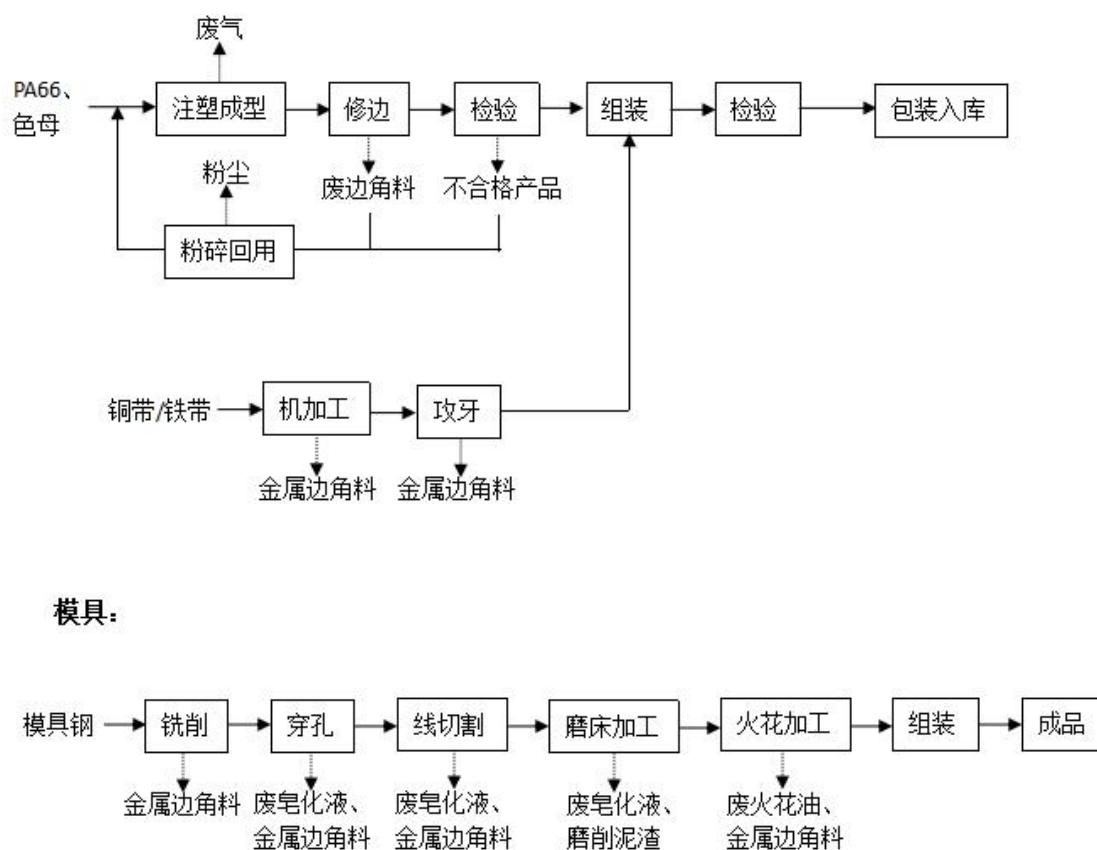
图 2-1 本项目生产工艺流程及产污节点图
