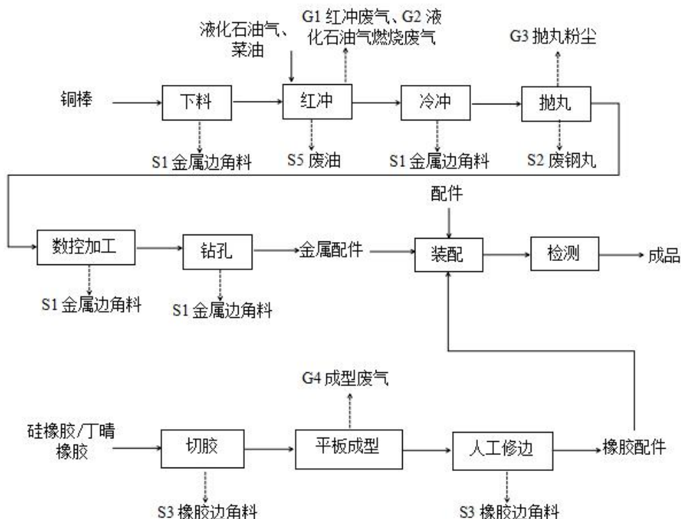
图 2-1 密封件生产工艺流程及产污节点图
