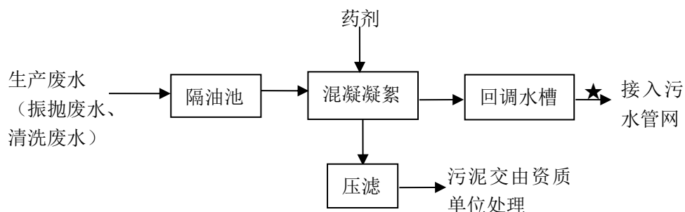
图 3-1 废水处理工艺流程图
