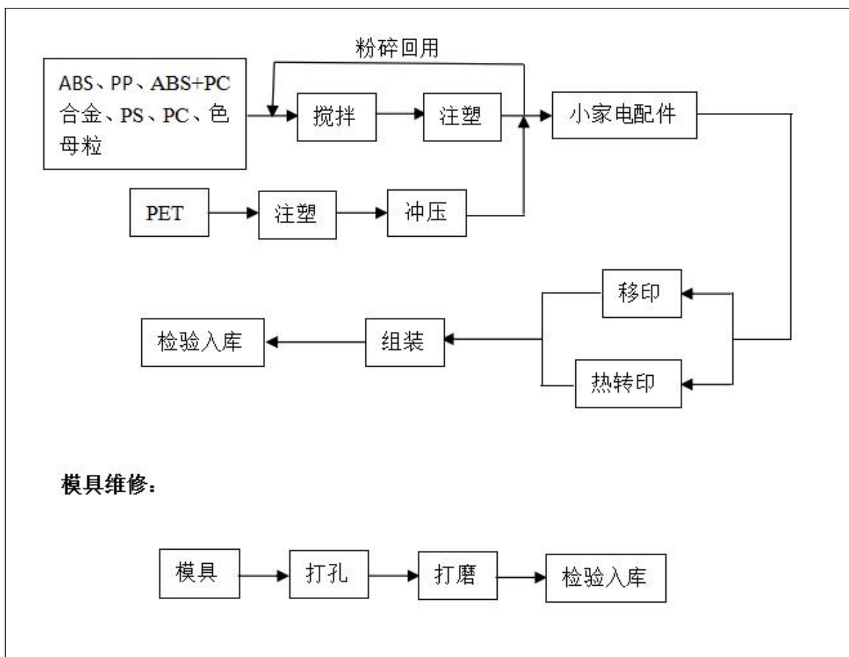
图 2-1 生产工艺流程及产污节点图
